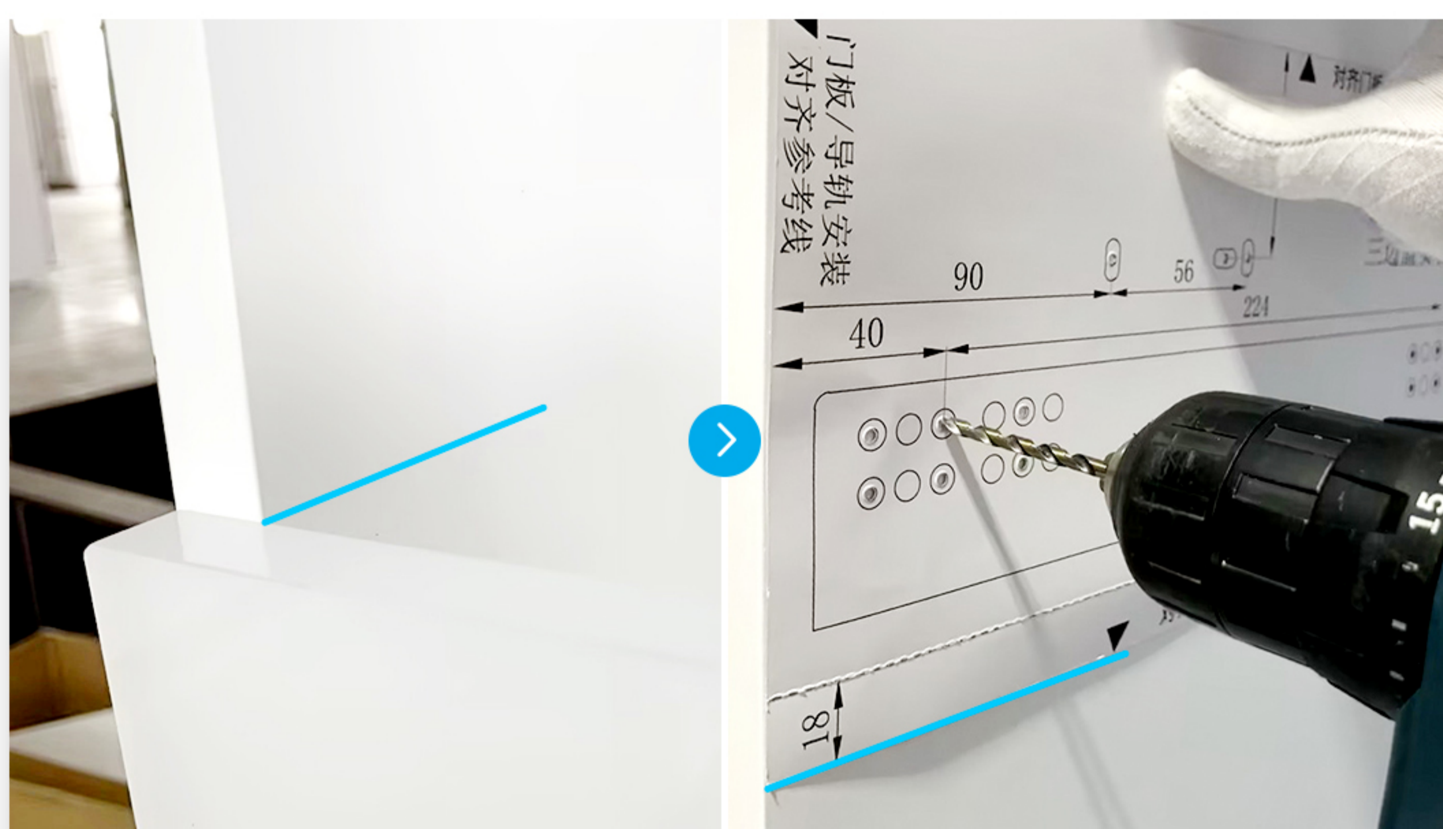
上层滑轨预钻孔 模板齐平面板顶线（左/右）
