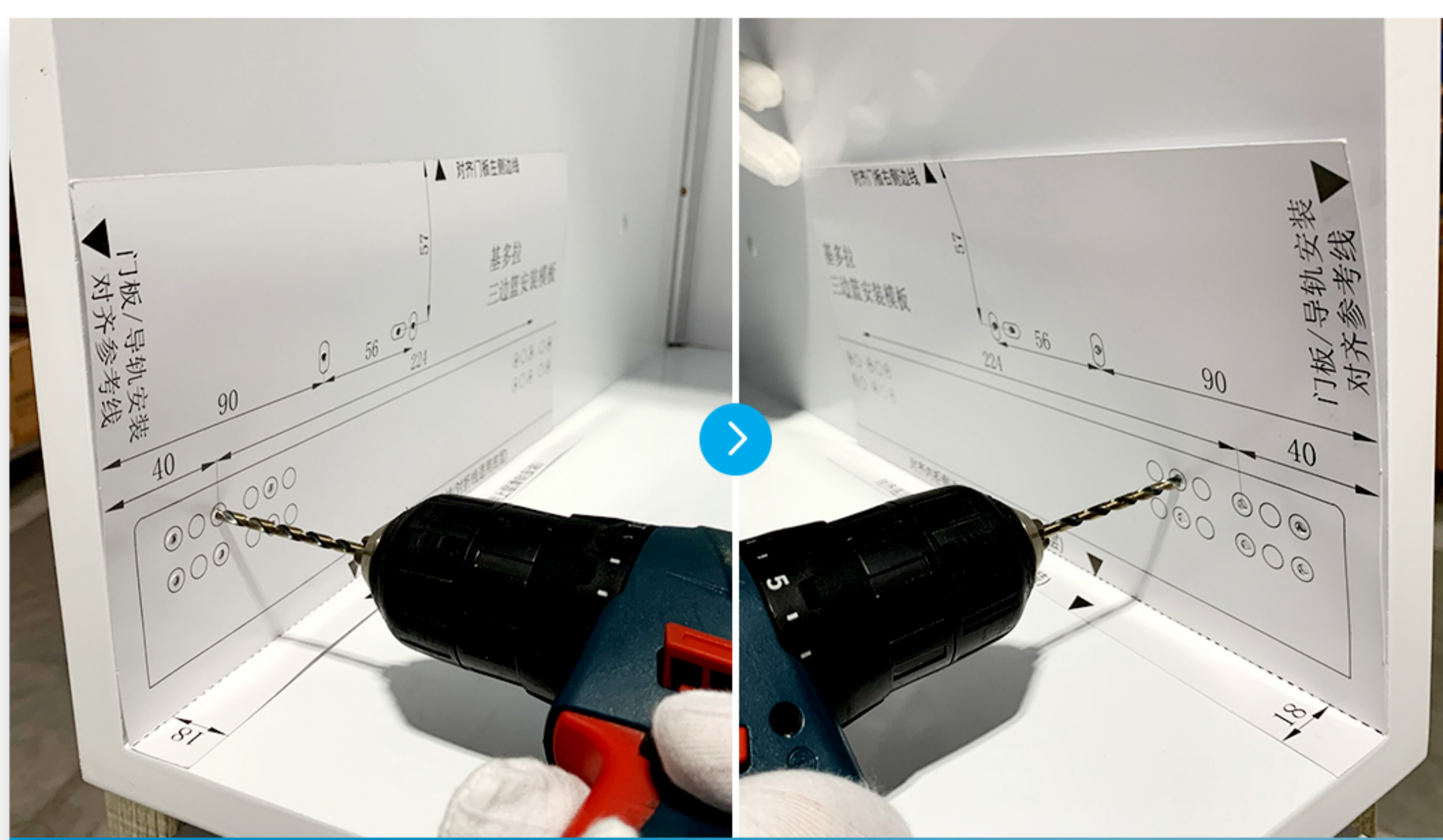
下层滑轨预钻孔 使用安装模板-折边对齐（左/右）
