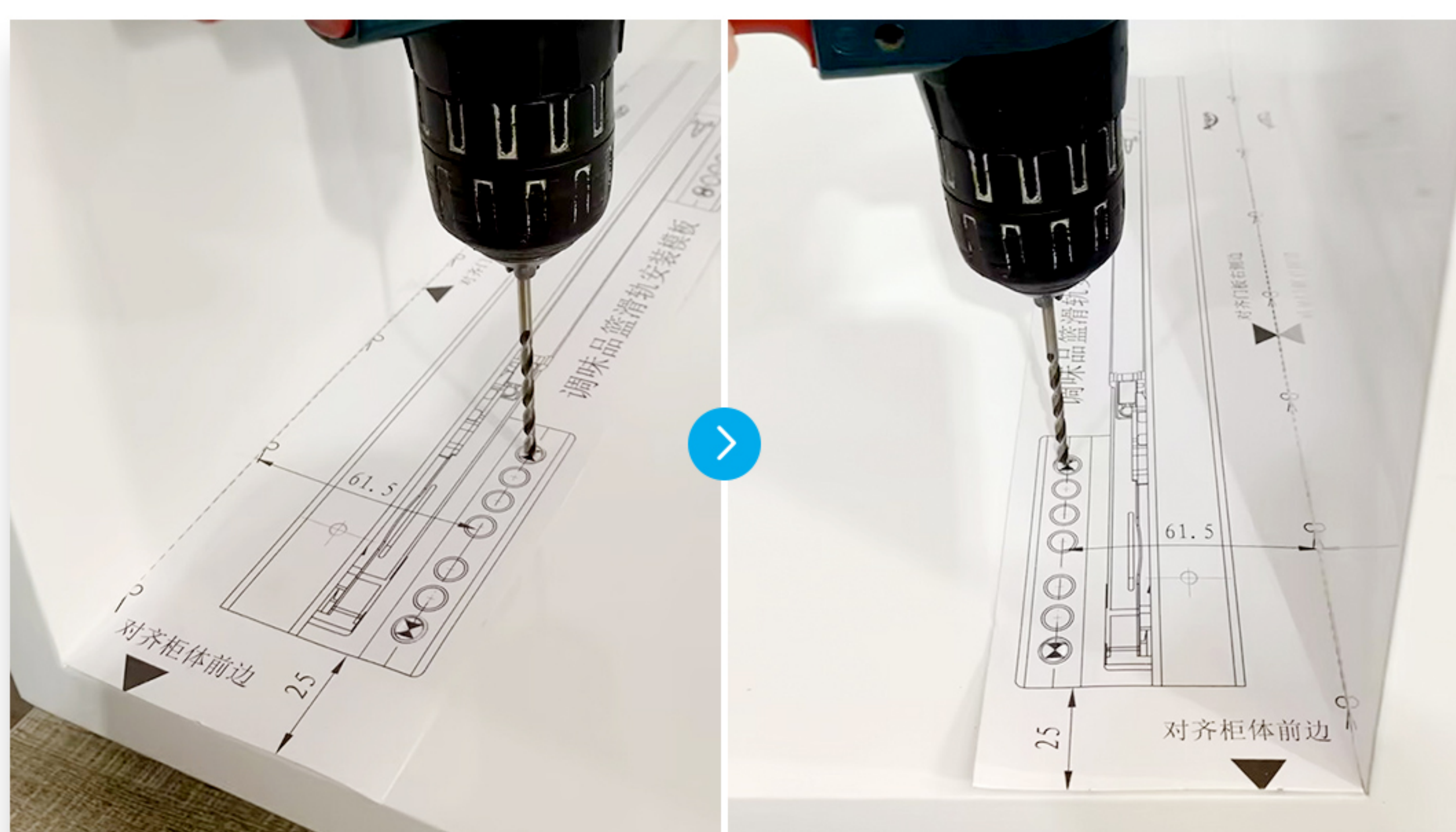
滑轨预钻孔 模板齐平面板顶线（左/右）
